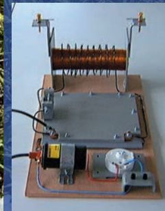
Nachbau eines Tesla-Trafos ca. 1996
